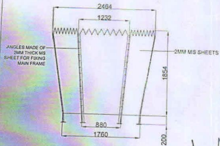
ELEVATION
